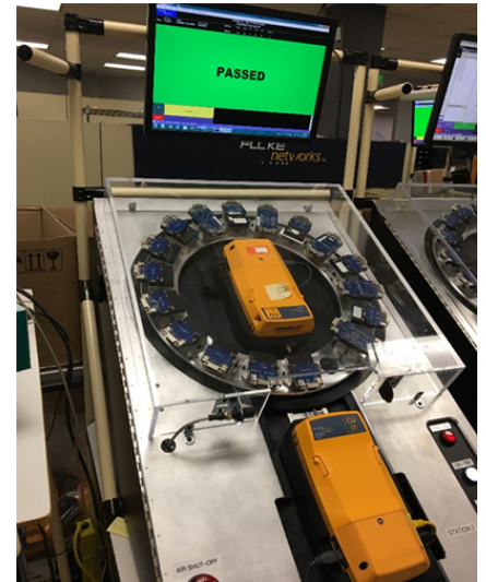
Figura 1: Estación de calibración de cobre. Diecisiete artefactos de diseño hechos a la medida están conectados en secuencia a la unidad Versiv para calibrarla. La configuración de rueda automatizada solo se usa en la fábrica para gestionar volúmenes de producción.
