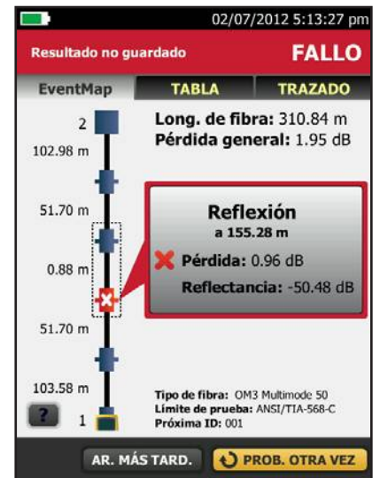
Vista EventMap con ayuda en pantalla
