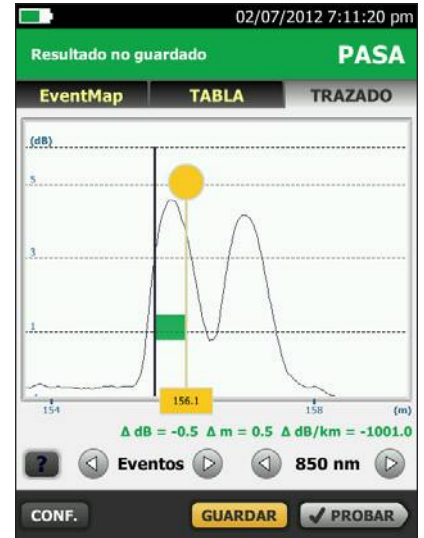
Zona muerta de eventos y atenuación extremadamente corta
