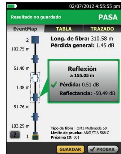
Vista gráfica EventMap
